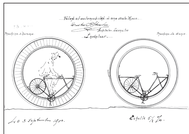
■ Eenwielige fiets van Gustave Strauven, 1900 ■ Vélopede automobile à une seule roue de Gustave Strauven, 1900 ■ One-wheel bike of Gustave Strauven, 1900 [Archistory Brussels]
