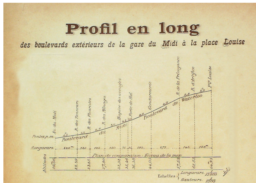
■ Hoogte -en hellingskaart: de belangrijkste Brusselse hellingen ■ Carte d'altitude et du degré de déclivité des principales montées à Bruxelles ■ Altitude and gradient map indicating the most important Brussels slopes, La Pédale Militaire [AMVB]
